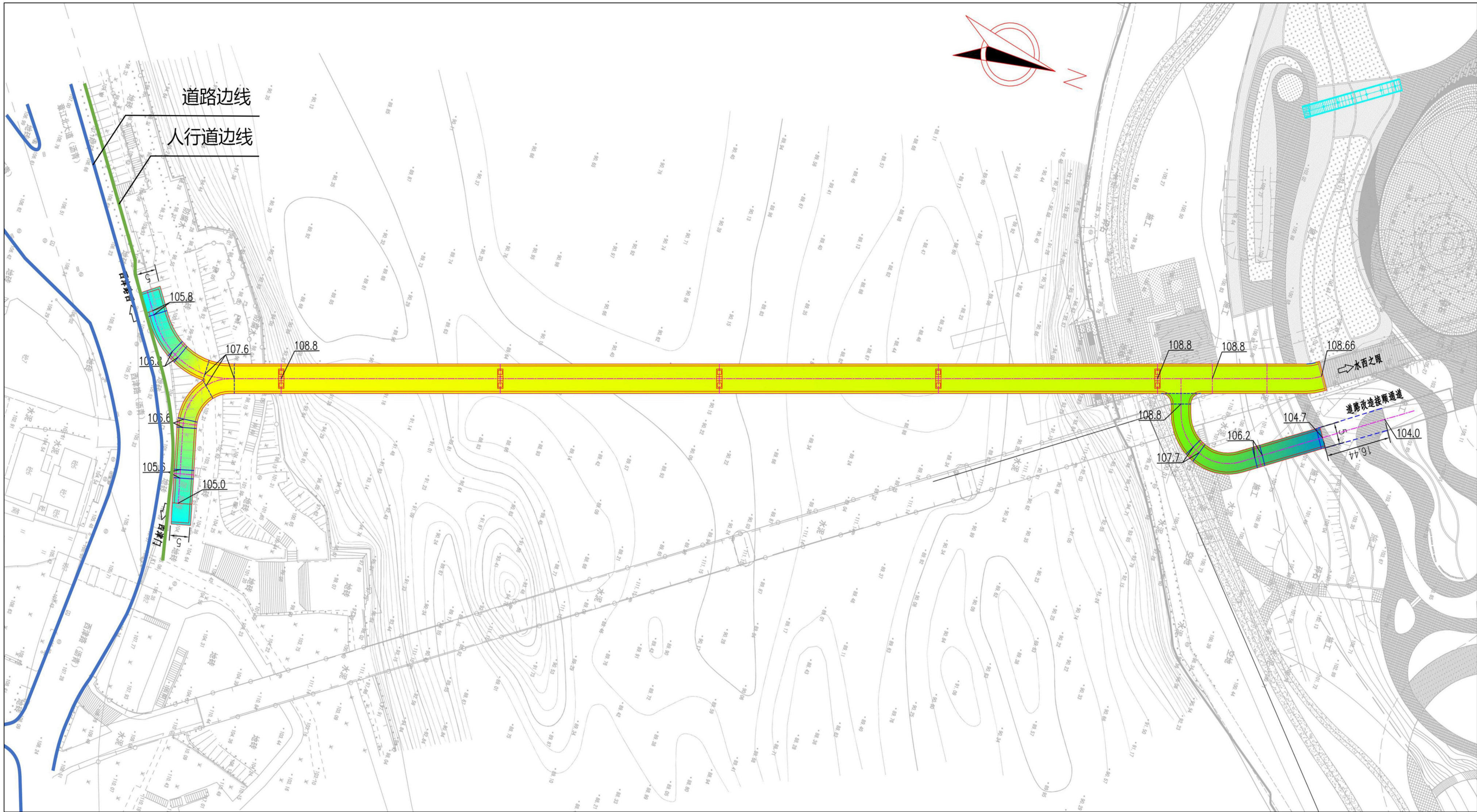
总平面图
